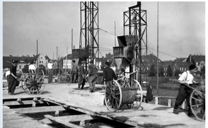
Holtz und Willemsen, Betonierarbeiten am Kesselhaus, 1936
